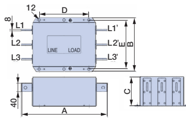
外形图 2
