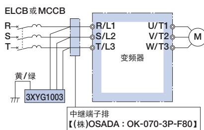
接线图
