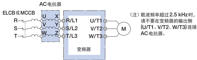
接线图
