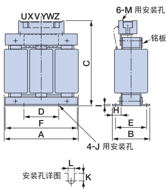
外形图 1
