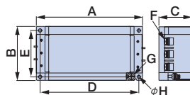
外形图 2
