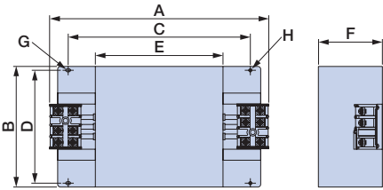
外形图 1
