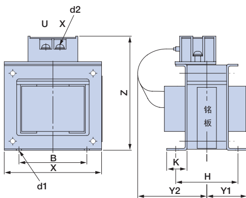
外形图 2
