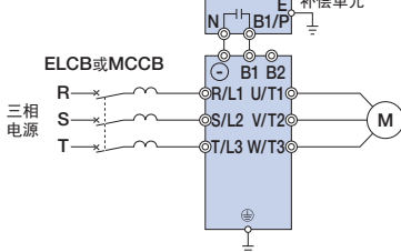
接线图
