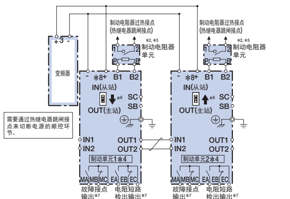
接线图 C
