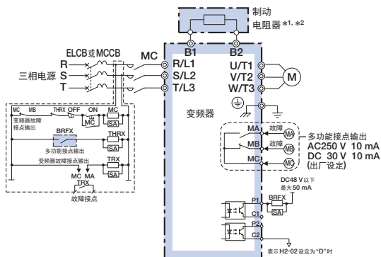
接线图A
