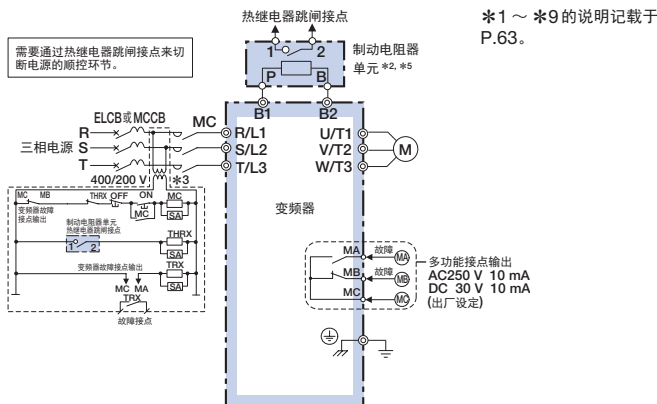
接线图 B
