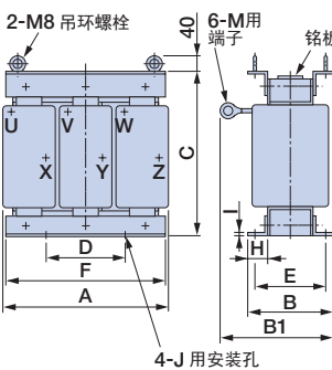
外形图2
