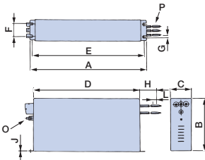
外形图 1
