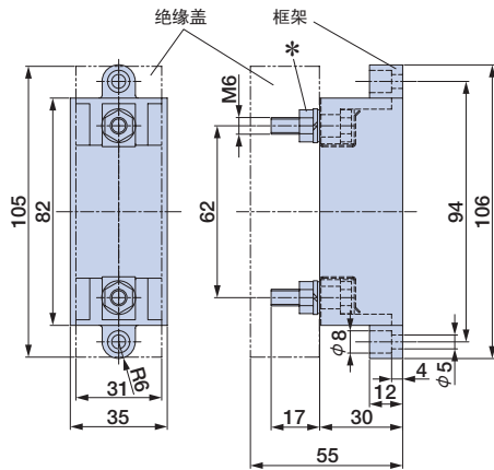
保险丝盒 外形尺寸 mm
