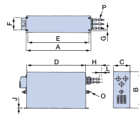
外形图 3
