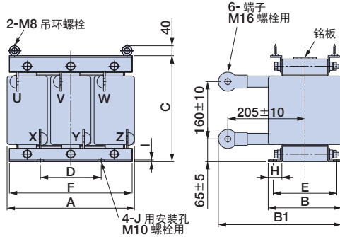
外形图3
