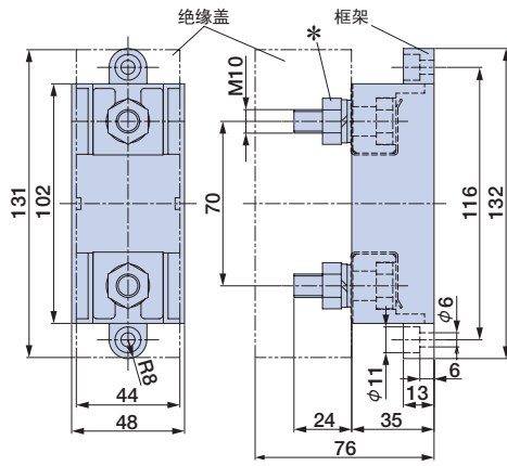
外形图 4
