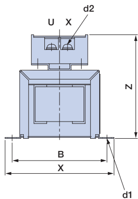
外形图 1
