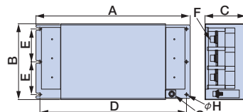
外形图 4
