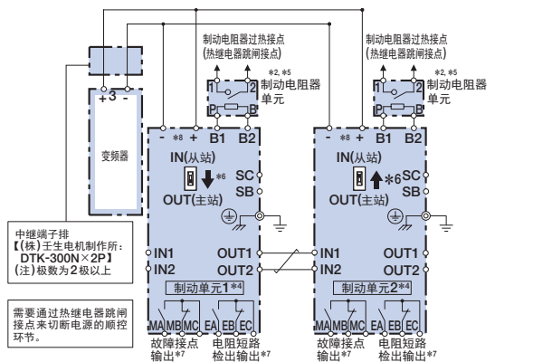
接线图 G
