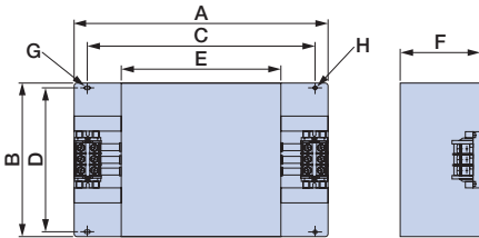
外形图 2
