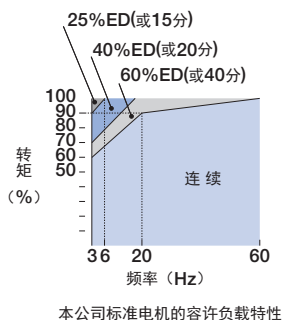
本公司标准电机的容许负载特性
