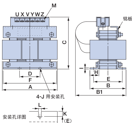
外形图 2
