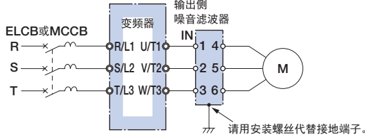
接线图
