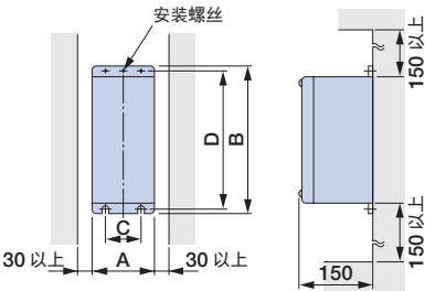
外形图 1
