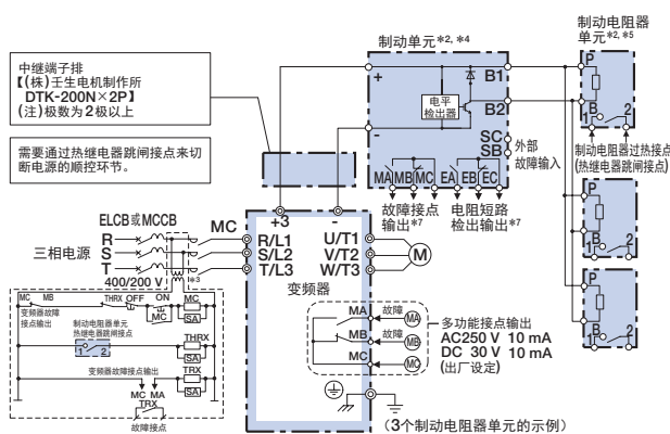
接线图 F
