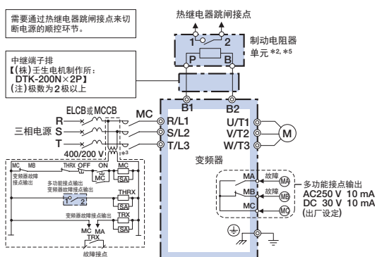
接线图 H
