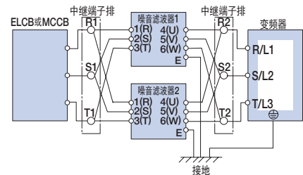
输入侧噪音滤波器及输出侧噪音滤波器的并联连接方法(2 个并联连接的示例)
