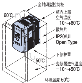
· 全封闭型控制柜内的安装图
