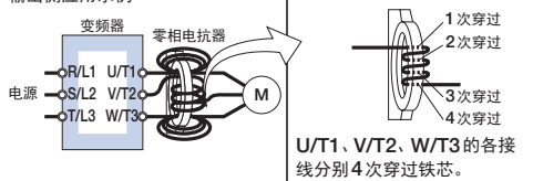
接线图a
