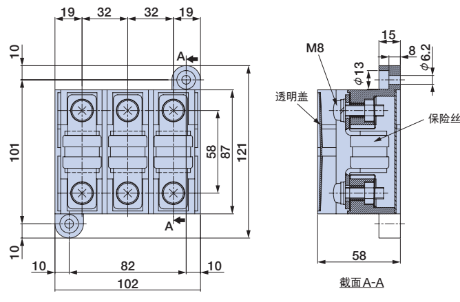
外形图2
