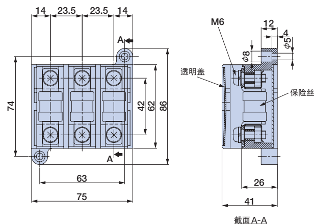
外形图1
