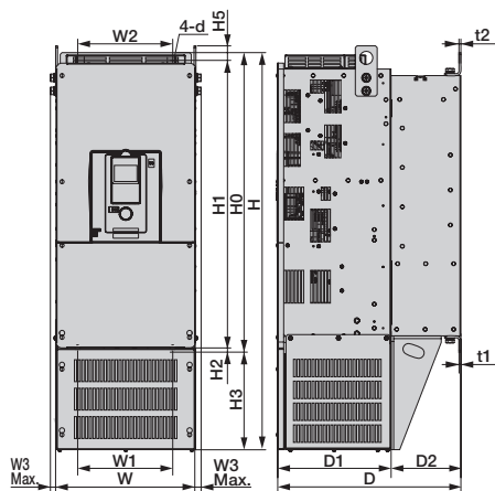
外形图 4
