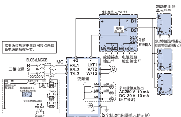
接线图D
