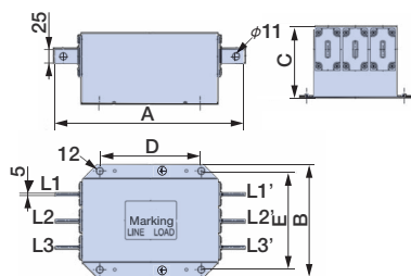
外形图 1
