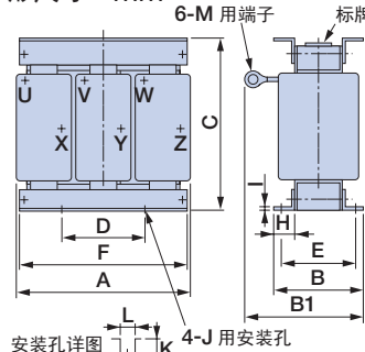
外形图1
