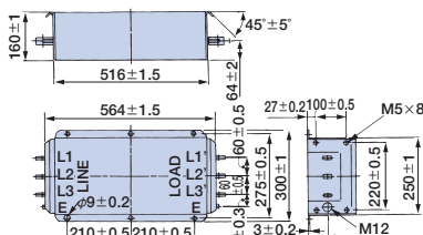
外形图 4
