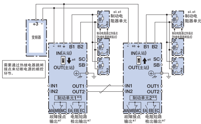
接线图 E
