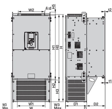
外形图 5
