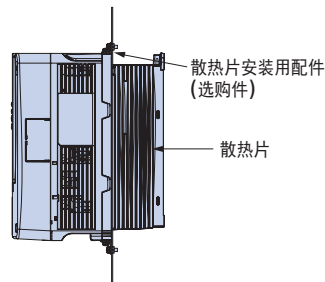
· 散热片外置安装图
